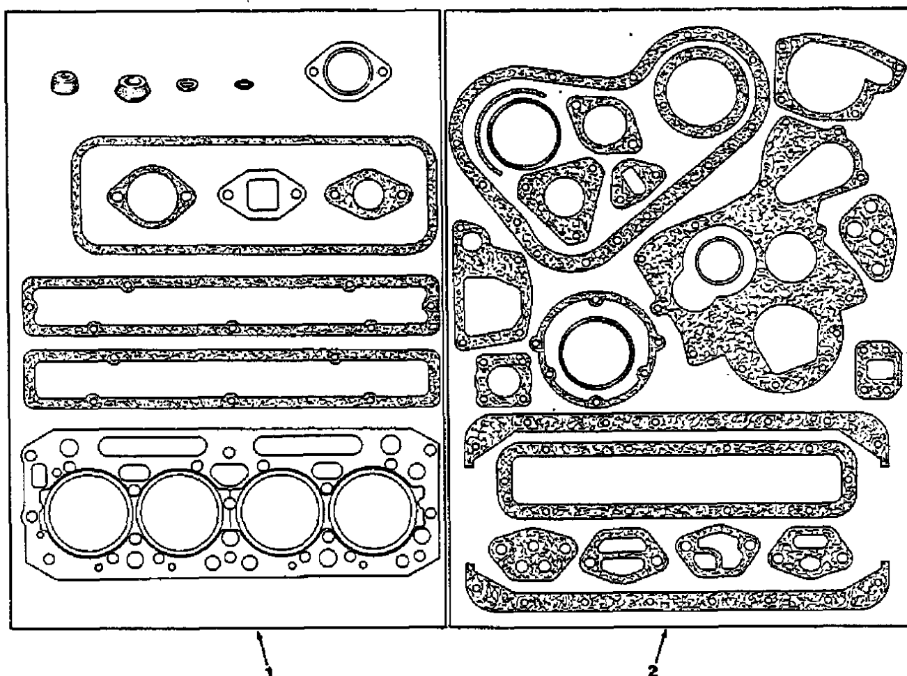
Fig. 17 - Gasket Kits
