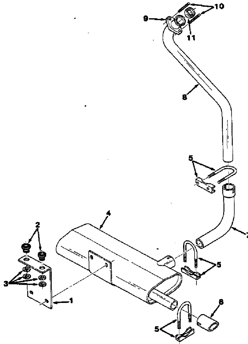
Fig. 19 - Muffler Group
