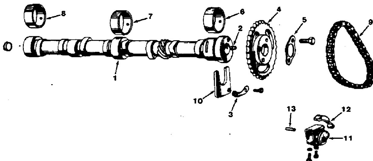
Fig. 4 - Camshaft Group
