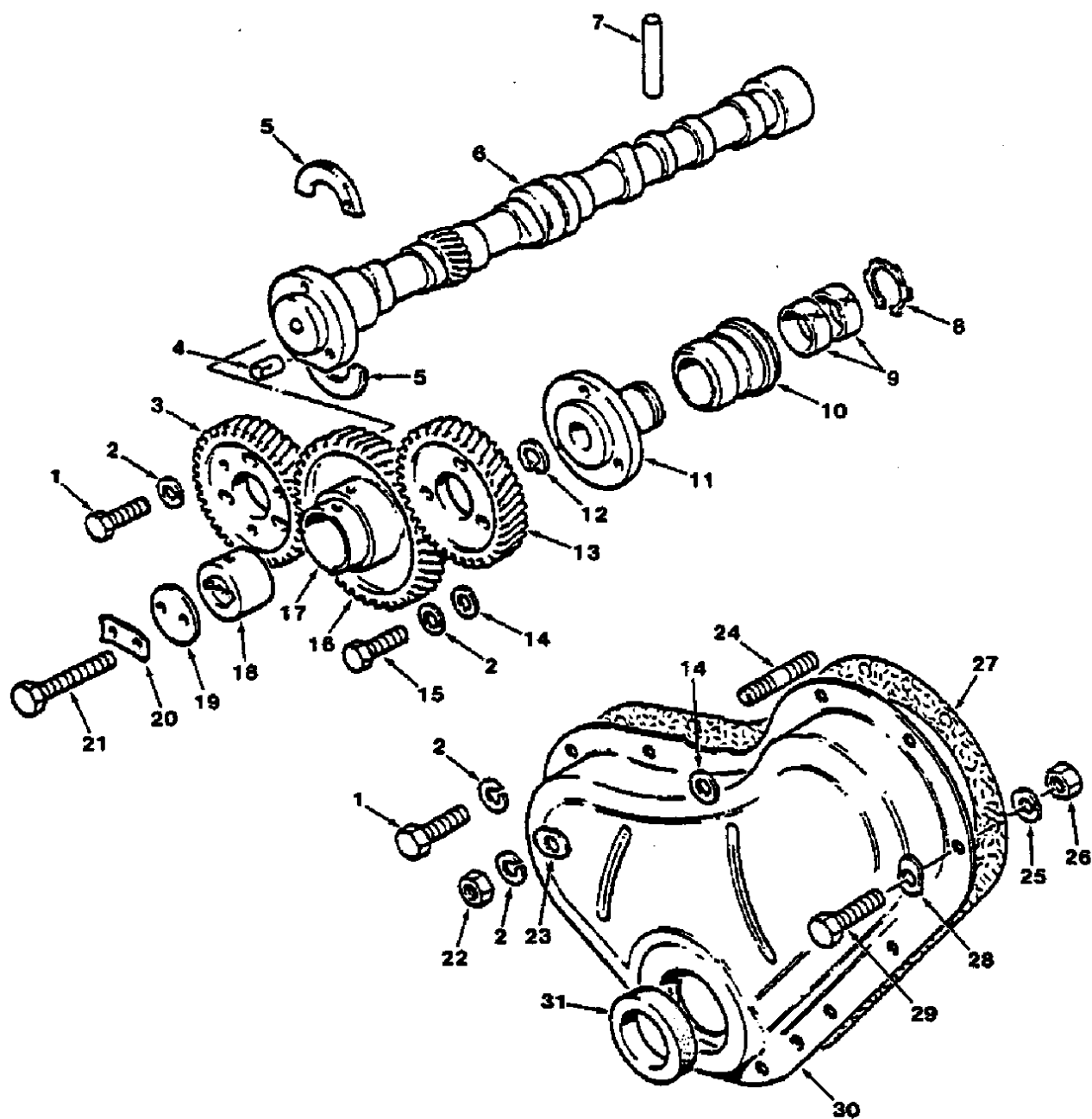
Fig. 5 - Camshaft Group
